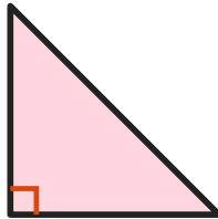
le triangle rectangle
