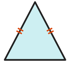
le triangle isocèle
