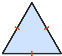
le triangle équilatéral
